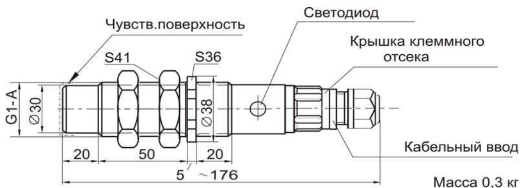
Рисунок 1 – Сигнализатор уровня
